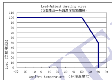
负载电流—环境温度降额曲线 (24V、36V 输出电压):
