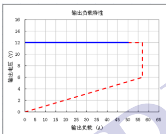
输出特性曲线图 (12V 输出电压):
