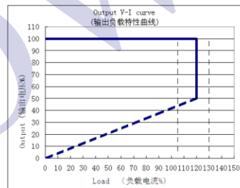
输出特性曲线图 (24V、36V 输出电压):
